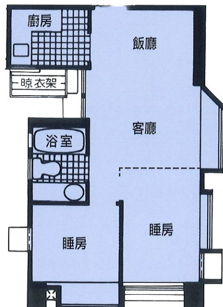
低層D, E單位 實: 370' 建: 508' - 521'
